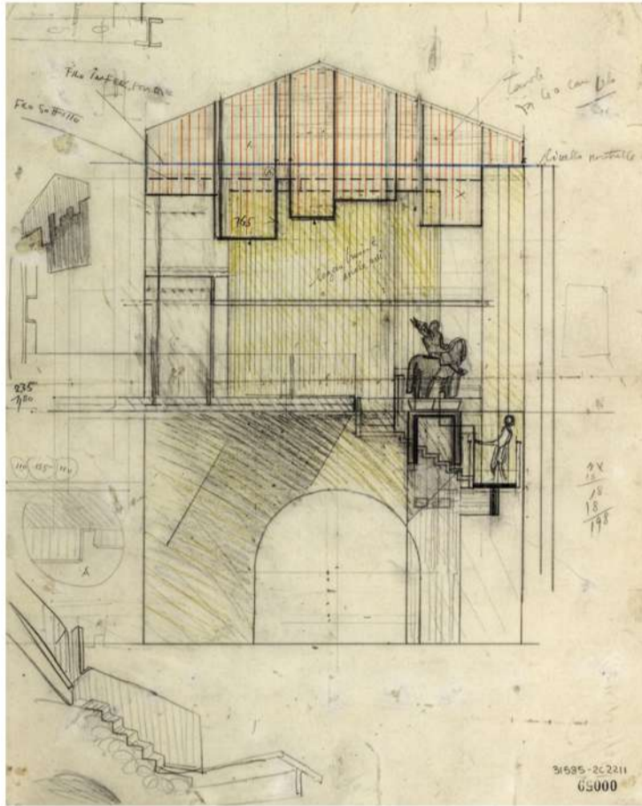
Carlo Scarpa. Museo de Castelvecchio. Verona
