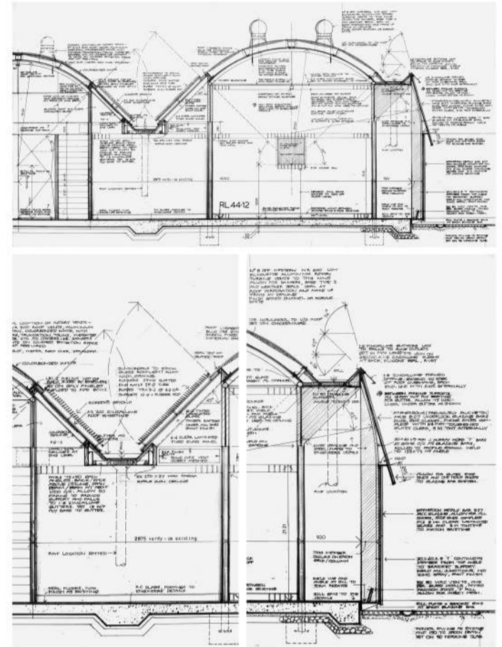
Glenn Murcutt. Museo Kempsey. Detalles dibujados a mano.
