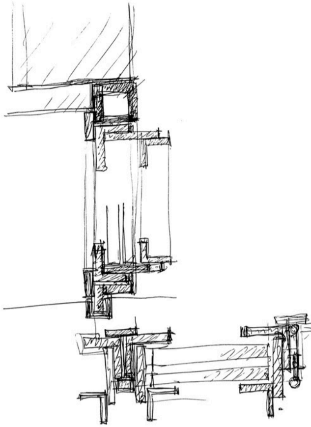
Eduardo Souto de Moura. Detalles de carpintería
