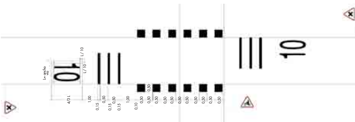
• Caso 3: señalización de cruce entre una vía ciclista con prioridad de paso y una vía motorizada de baja intensidad de tráfico o con una vía peatonal.
