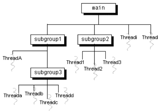
Figura 6.3. Representación de los grupos de Threads.
