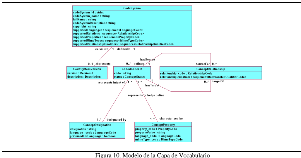
Figura 10. Modelo de la Capa de Vocabulario
