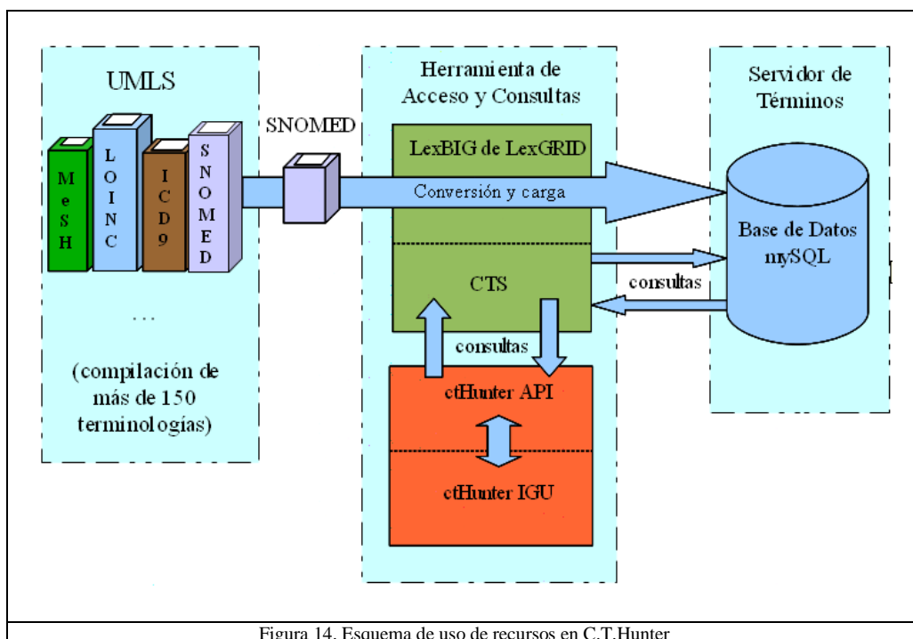
Figura 14. Esquema de uso de recursos en C.T.Hunter
