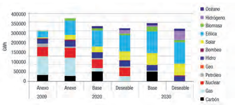
Figura 6. Producción de electricidad.
