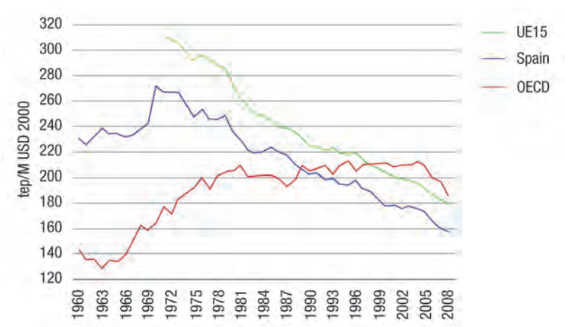
Figura 3. Evolución de la intensidad energética. (Fuente: Agencia Internacional de la Energía, 2009).
